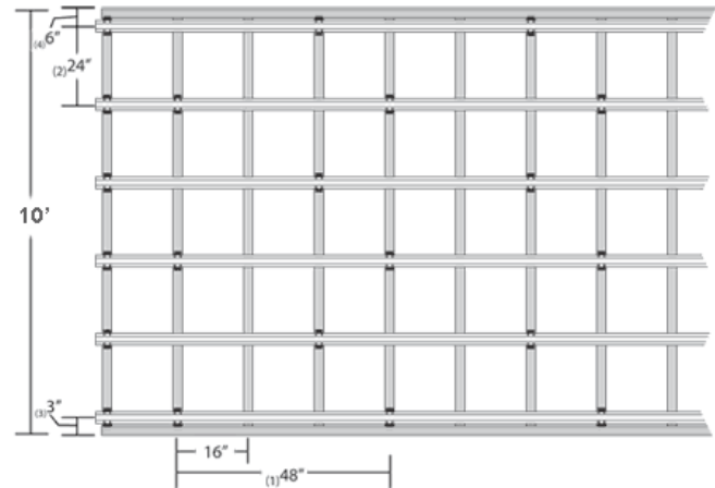
Patrón de disposición para los clips de insonorización Green Glue
